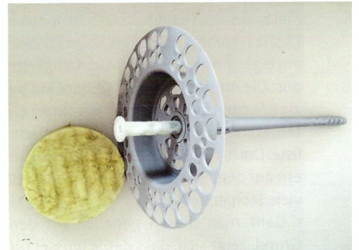
Der versenkbare Schraubdübel speziell für Mineralwolle WDVS-Systemdämmplatten.
